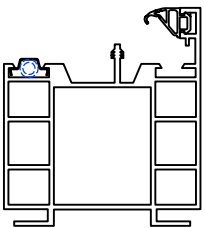
Cheminement Câbles traverse haute (Vérins + Verrou)
